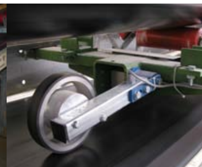
Robustes Messrad
